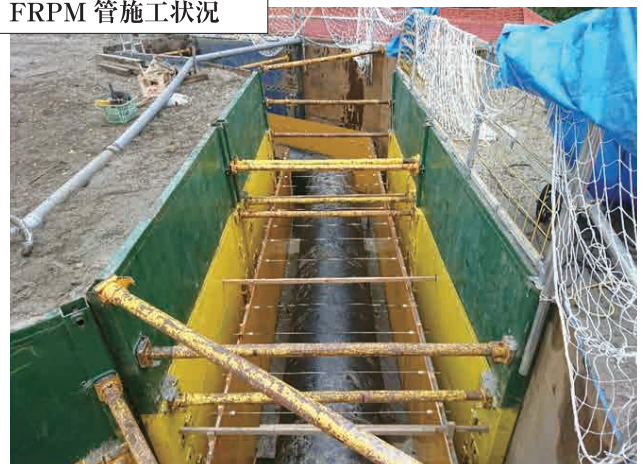
支線用水路6 FRPM管施工状況
